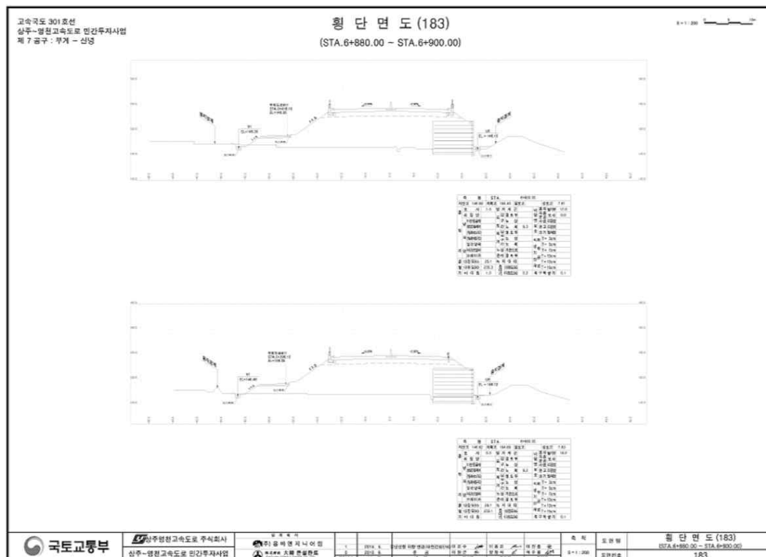
【그림 11.1.7】 단면도
